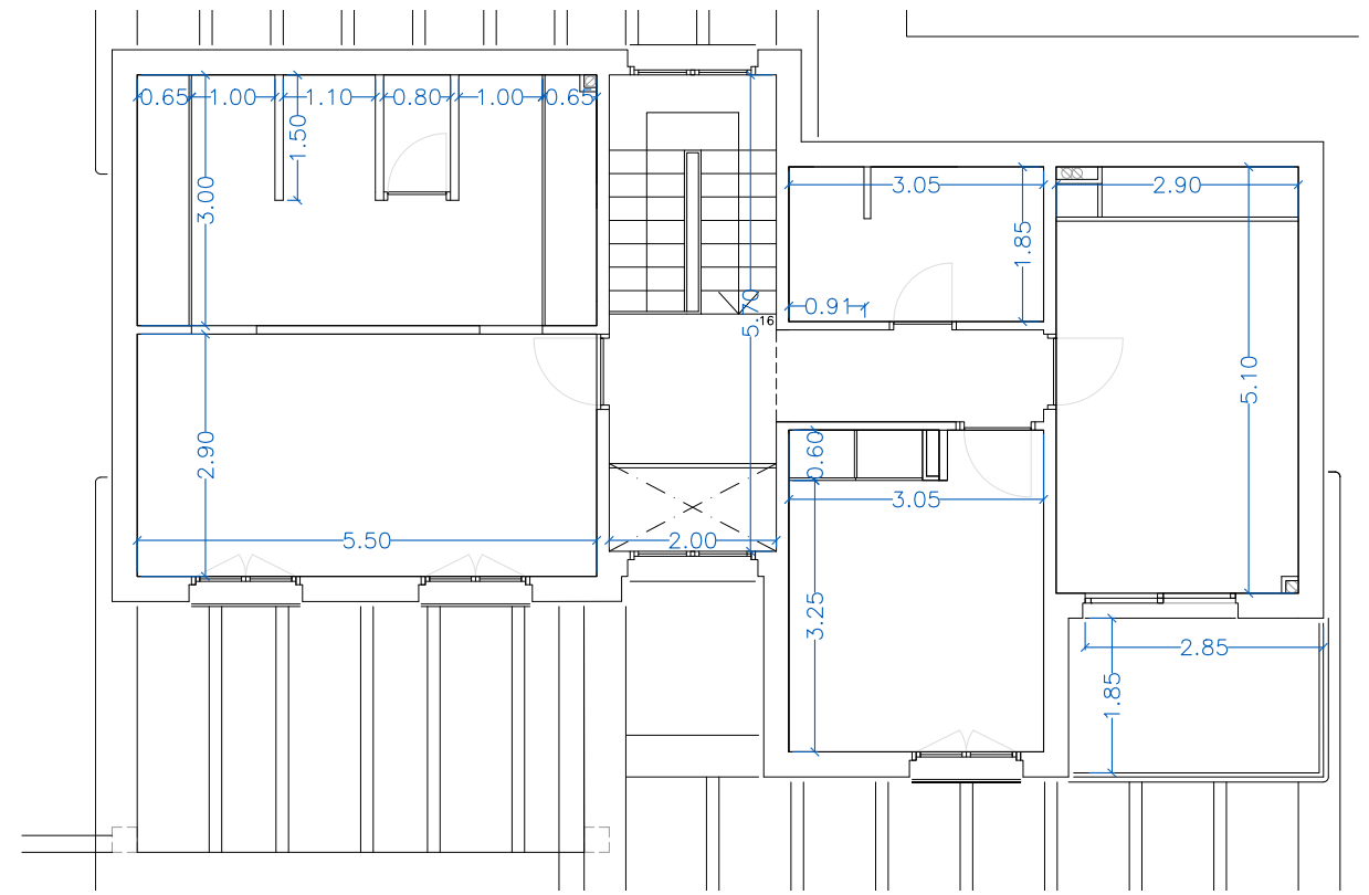
PLANTA PRIMERA
