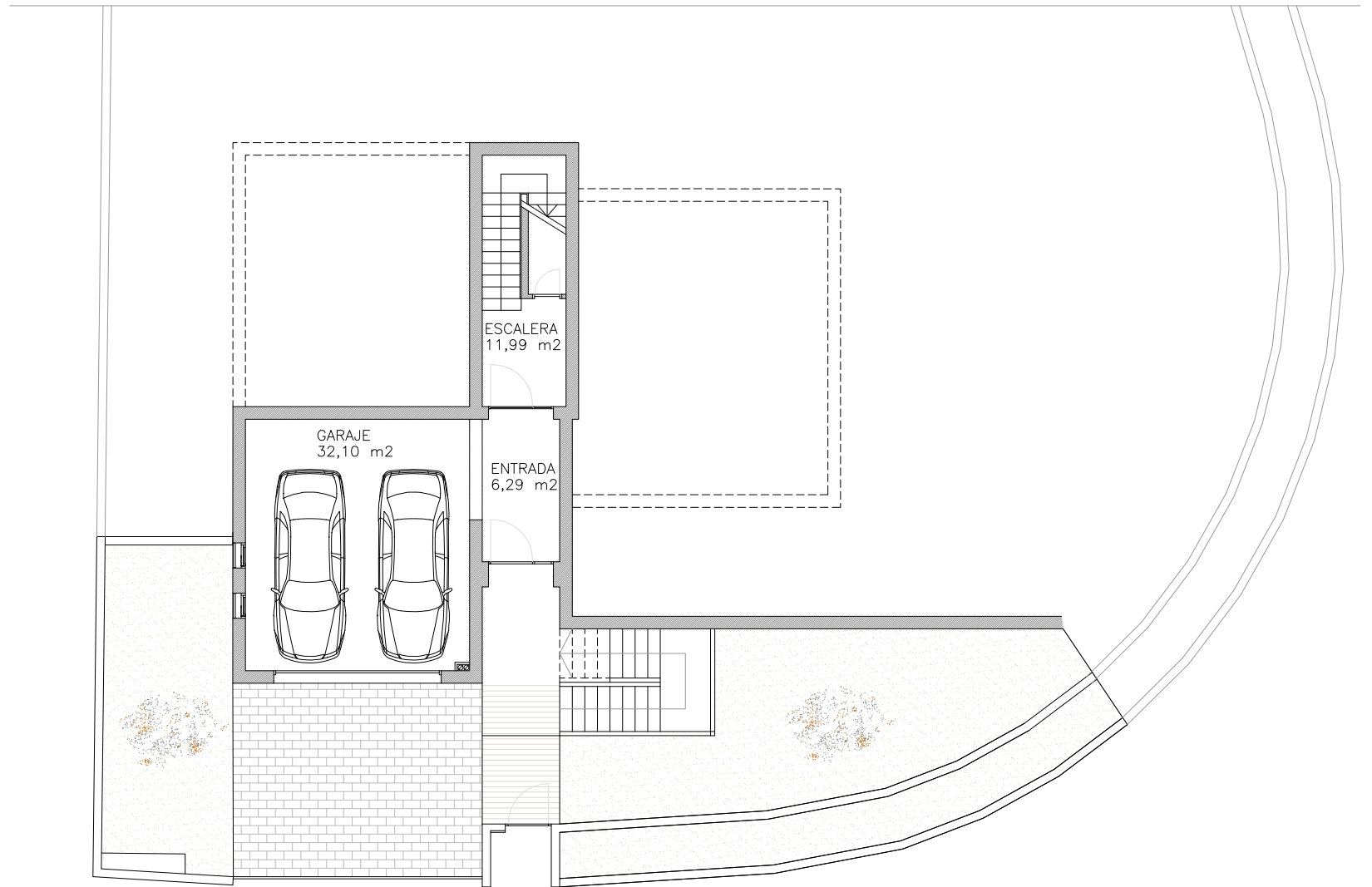
PLANTA SÓTANO
