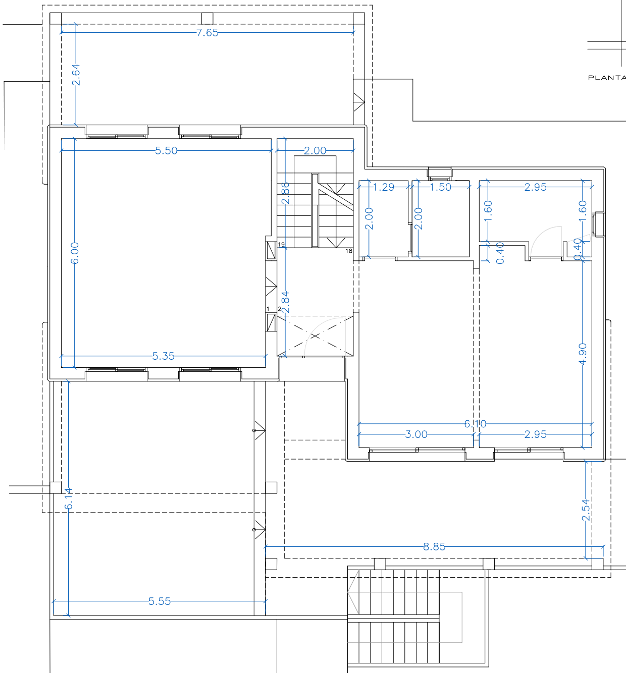
PLANTA BAJA
