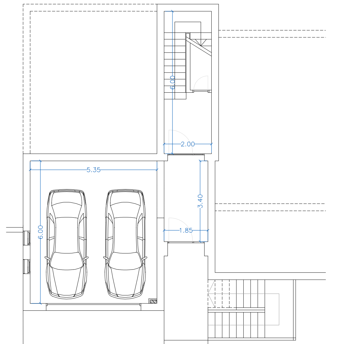
PLANTA SÓTANO
