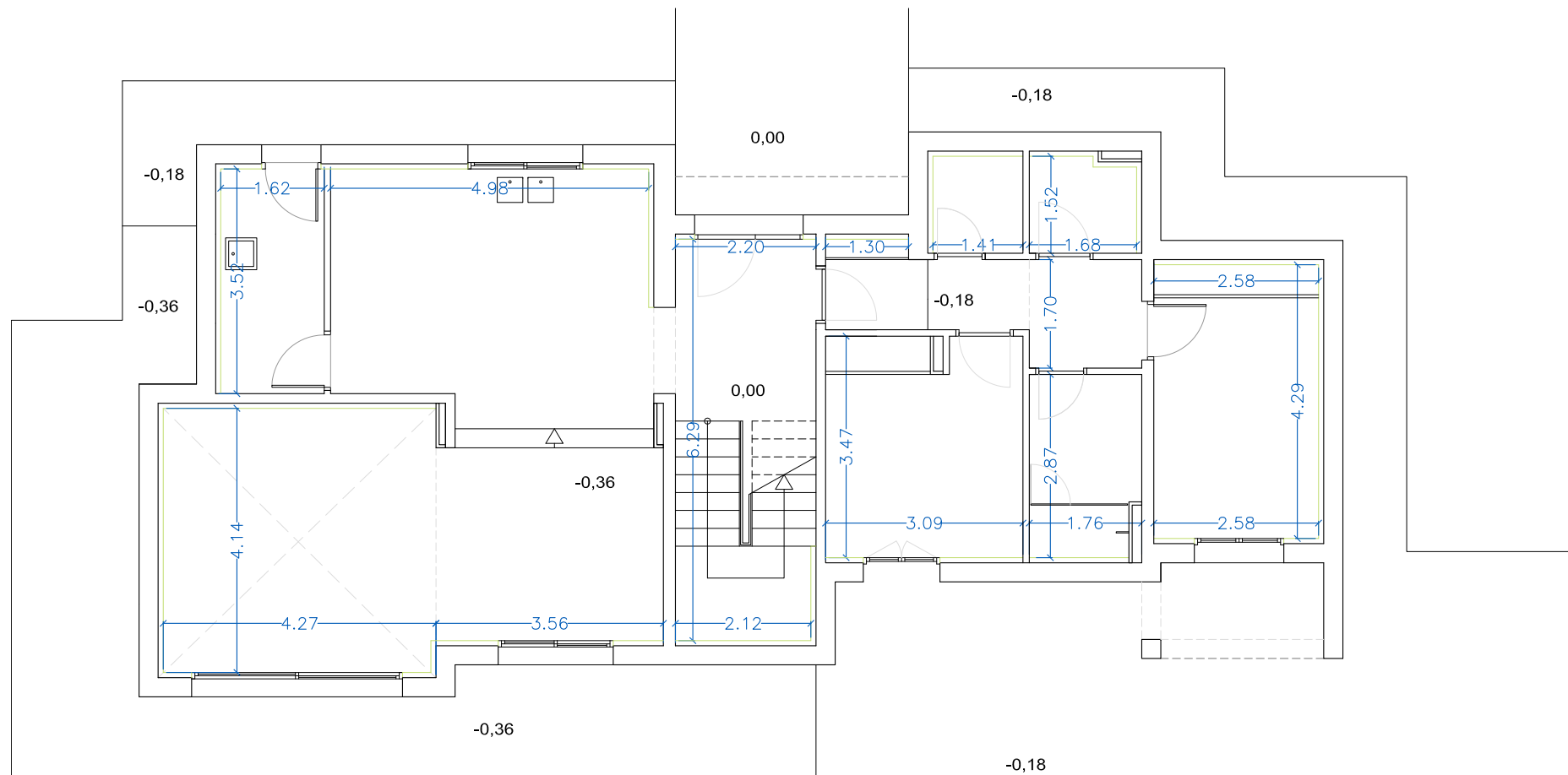
PLANTA BAJA
