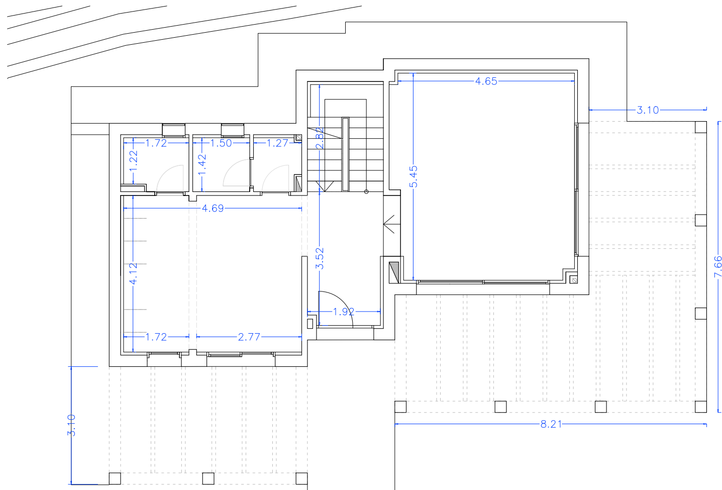
PLANTA BAJA
