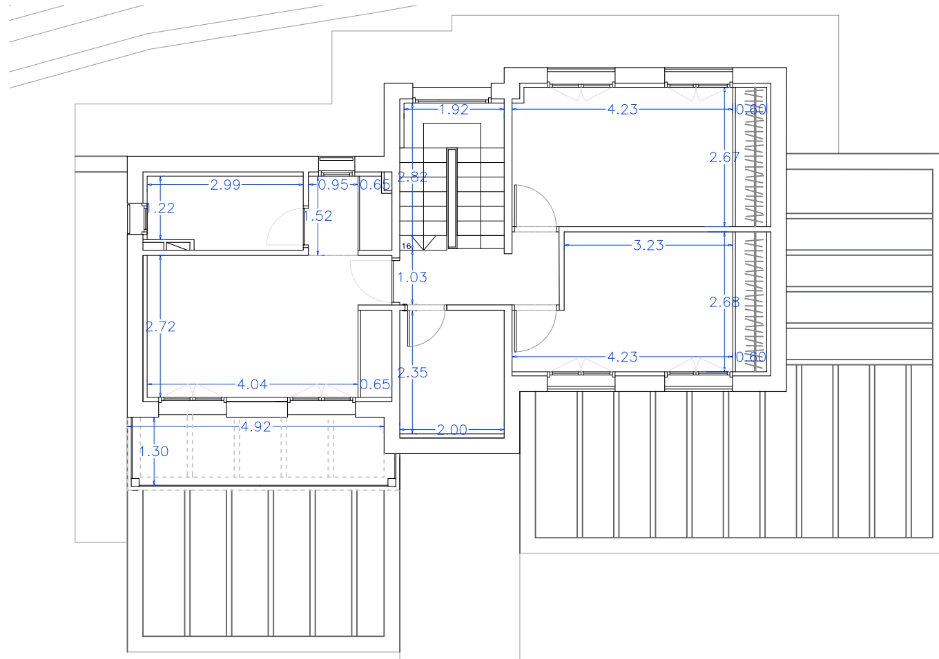
PLANTA PRIMERA
